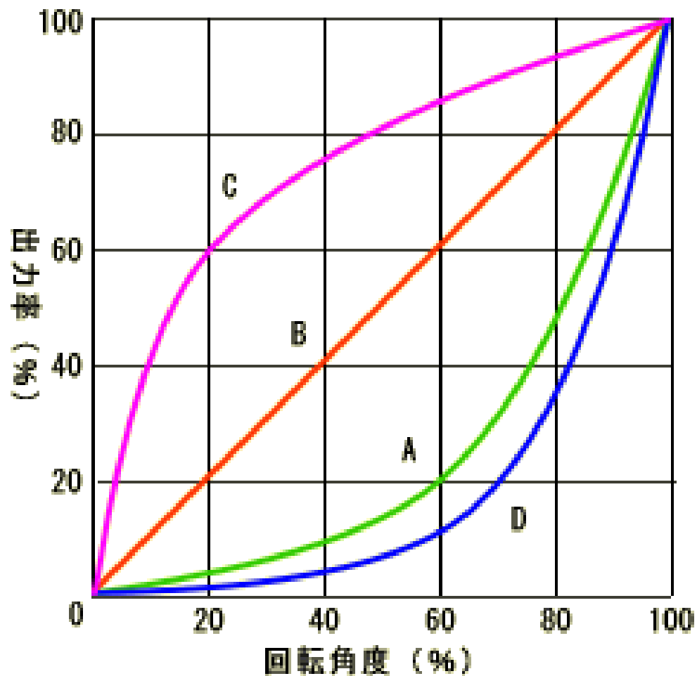
可変抵抗のカーブ率表
